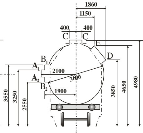
НАПРЕЧЕН РАЗРЕЗ
