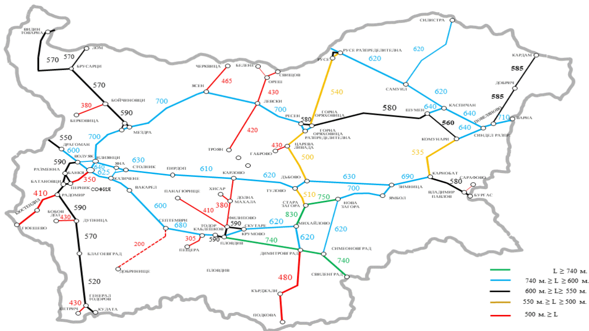
Карта на нормите за дължини на влаковете по участъци за движение без допълнителни условия
